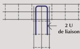
Détail liaisons angles
